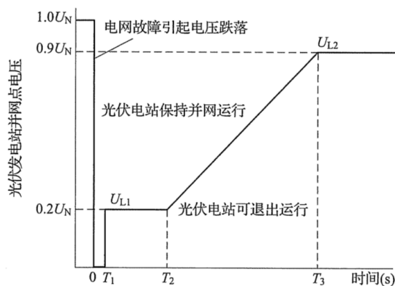
图 9.2.4 大、中型光伏电站低电压穿越能力要求
